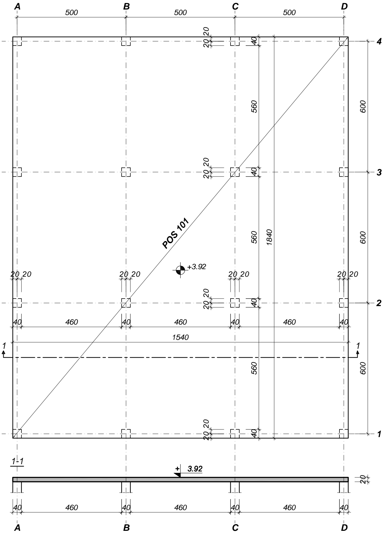
PRIMER P05 - List br.1 PLAN OPLATE KONSTRUKCIJE NA KOTI +3.92
