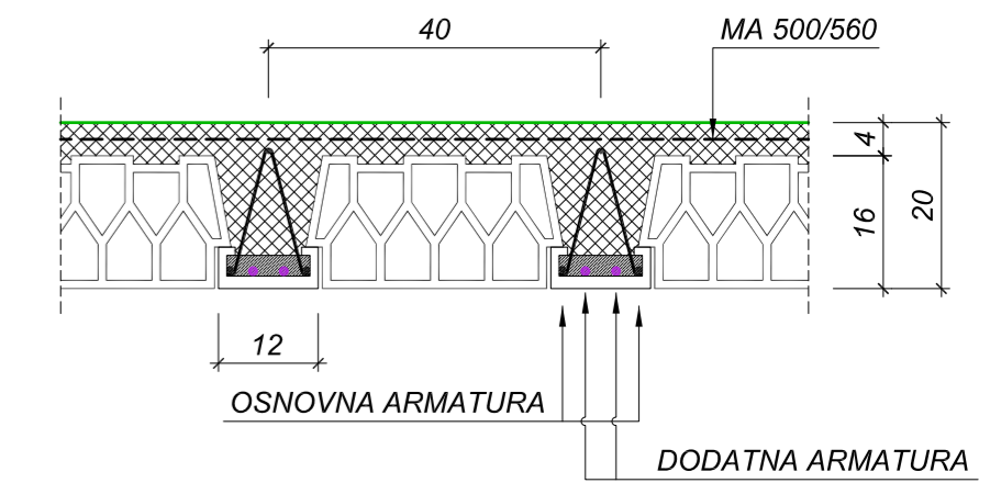
SPECIFIKACIJA LMT NOSAČA
