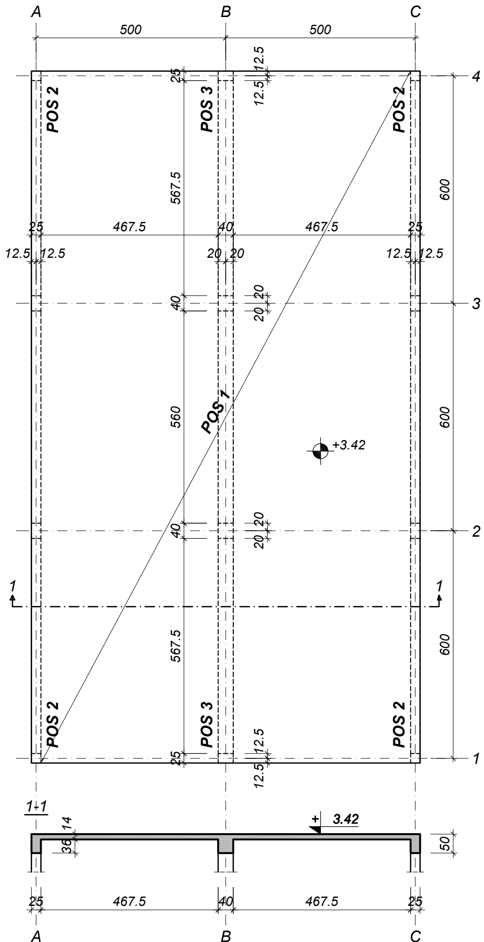
PRIMER P01 - List br.1 PLAN OPLATE KONSTRUKCIJE NA KOTI +3.42 VARIJANTA 1 (ploča u jednom pravcu)
