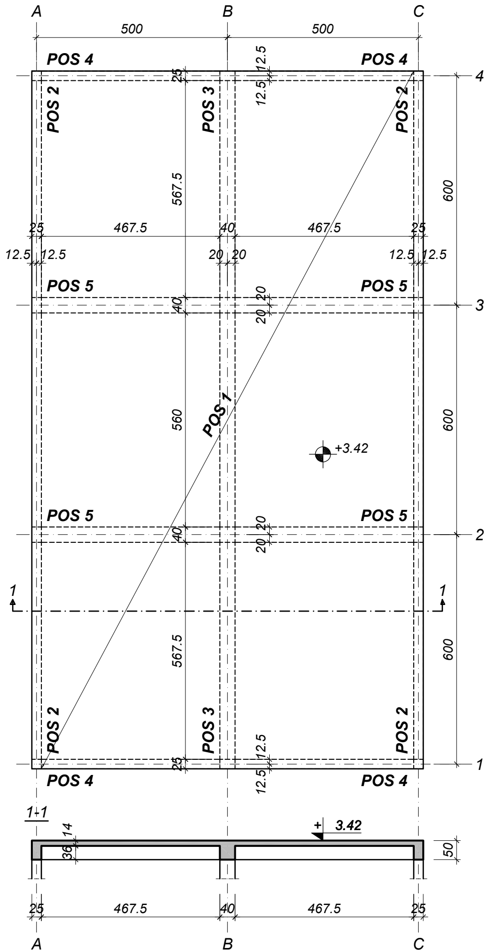
PRIMER P03 - List br.1 PLAN OPLATE KONSTRUKCIJE NA KOTI +3.42 VARIJANTA 2 (krstasta ploča)
