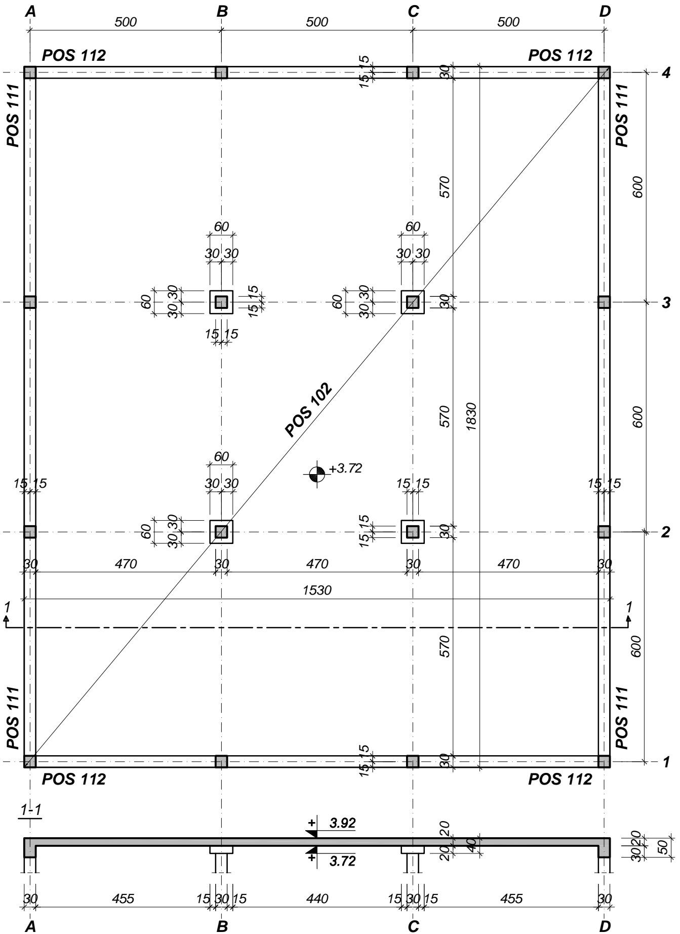
PRIMER P06 - List br.1 PLAN OPLATE KONSTRUKCIJE NA KOTI +3.92
