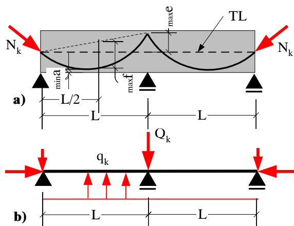
Slika 2.10 Trasa kabla sa maksimalnim ekscentricitetom i strelom
