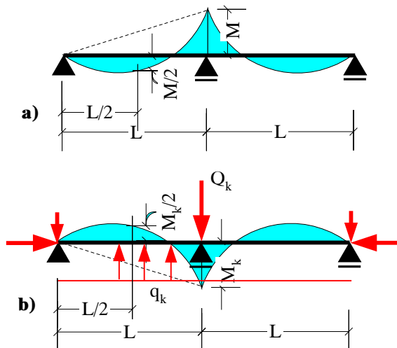
Slika 2.9 Momenti savijanja kontinualnog nosača
