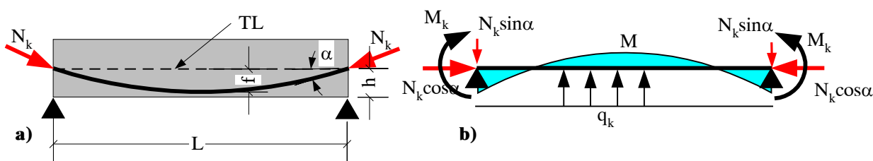
Slika 2.3 Efekat blokade pomerljivog oslonca proste grede
